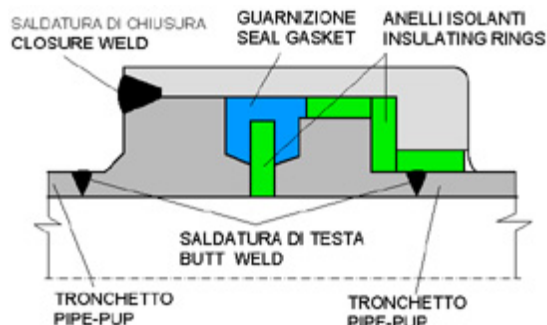
Sezione tipica del giunto isolante di linea - DN > 18" PN>25
